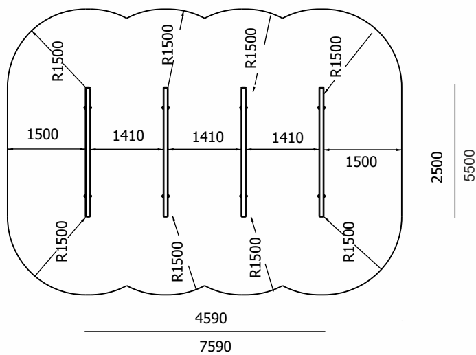
rzut poziomy ze strefą bezpieczeństwa skala 1:100
