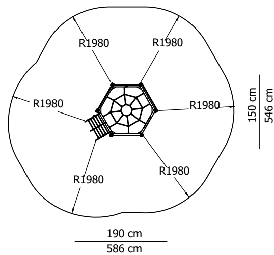
rzut poziomy ze strefą bezpieczeństwa skala 1 : 100
