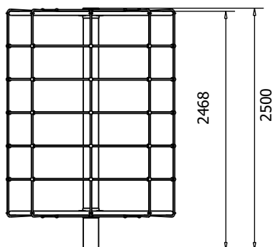
rzut pionowy
